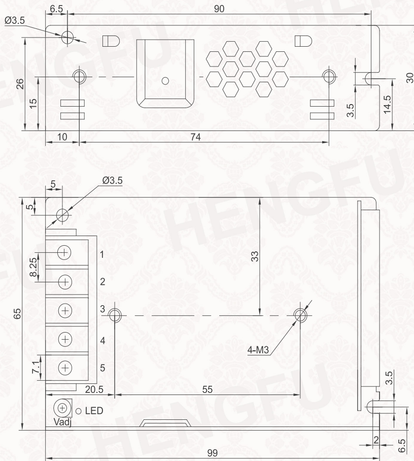
机壳 Frame
